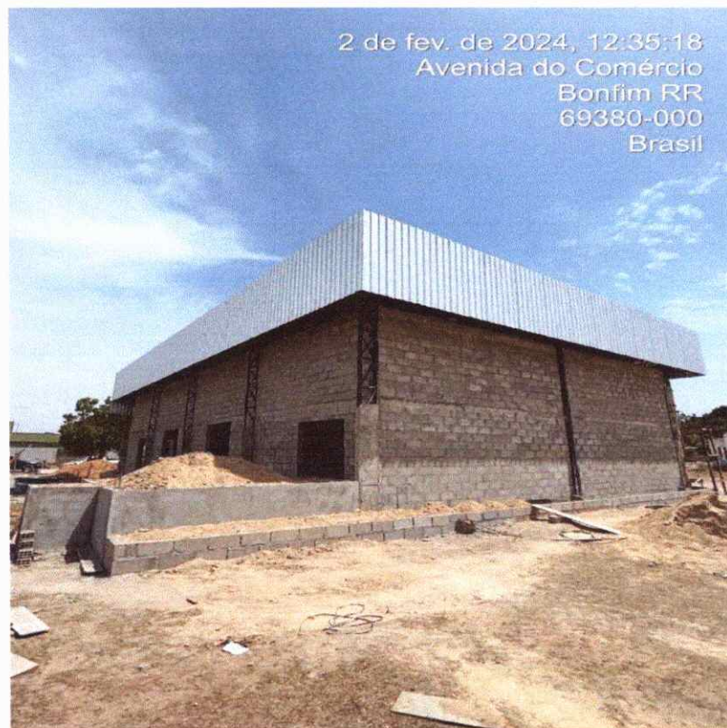
Figura 4: fechamento lateral com telha metálica
