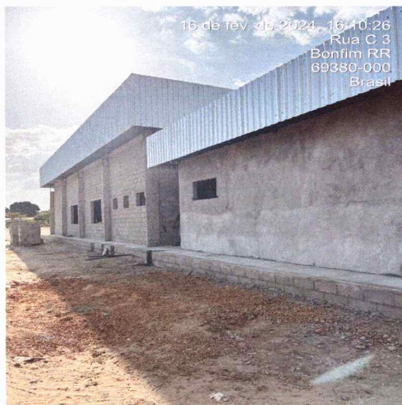
Figura 20: estrutura metálica para fechamento lateral
