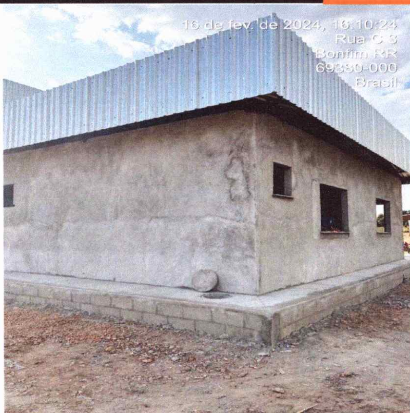
Figura 23: estrutura metálica da parte administrativa
