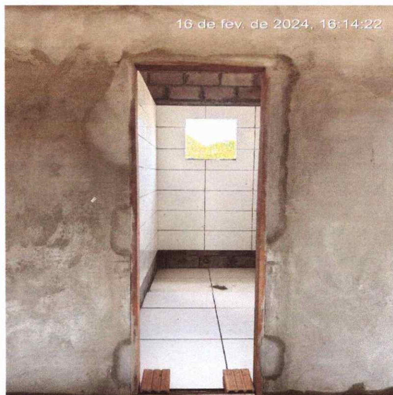
Figura 34: revestimento cerâmico parede e piso dos banheiros do galpão
