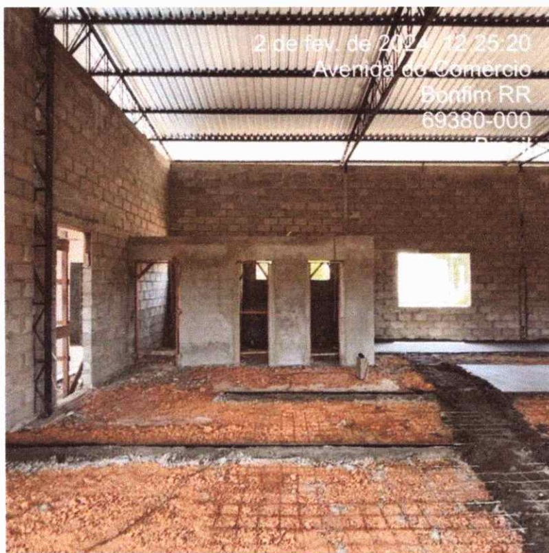
Figura 10: piso em concreto armado do galpão
