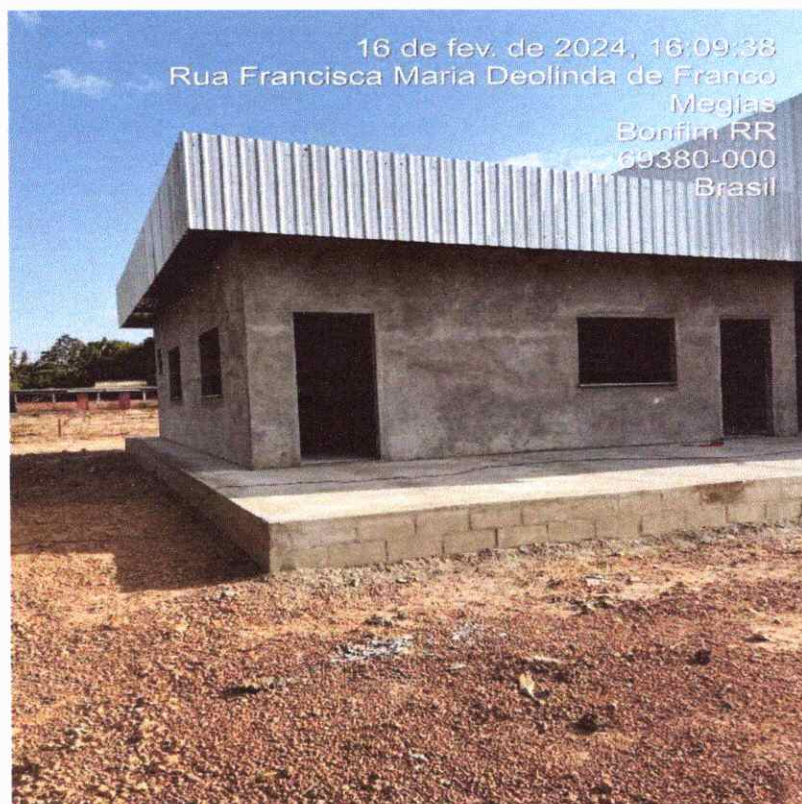
Figura 18: fechamento lateral em telha metálica
