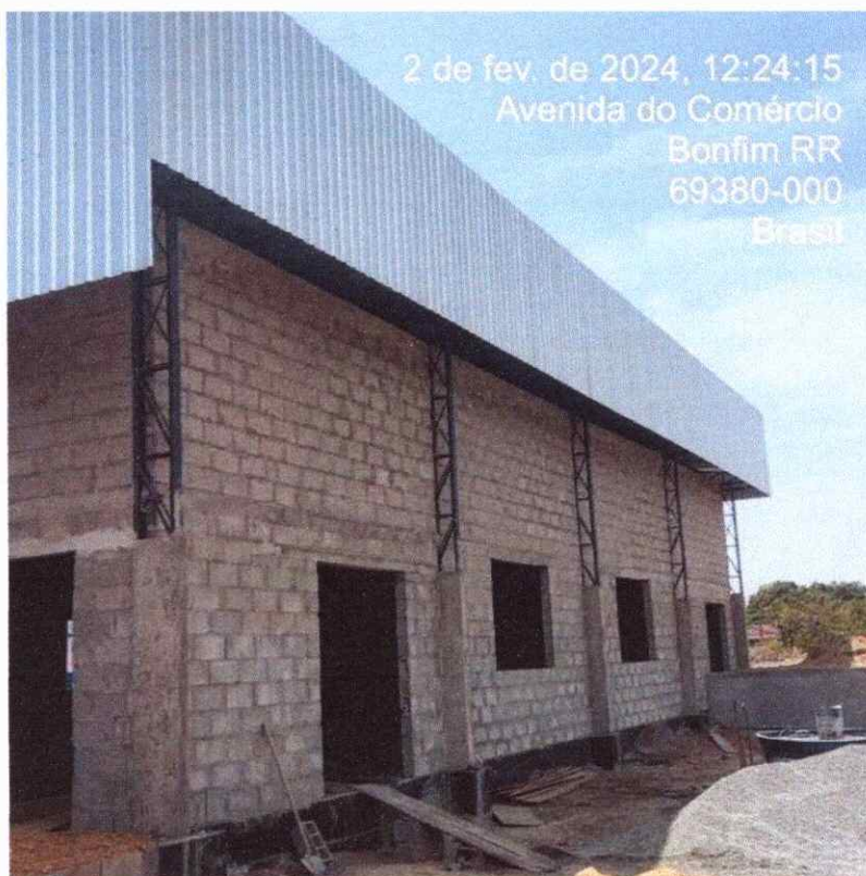
Figura 2: fechamento lateral com telha metálica
