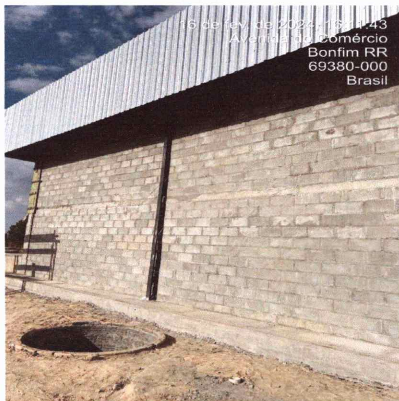
Figura 16: alvenaria de vedação em bloco de concreto
